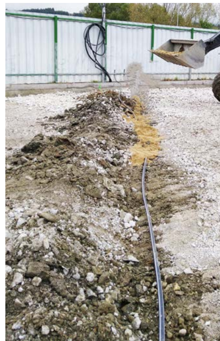
Napojenie objektu na sieť NN pomocou káblového vedenia v zemi
